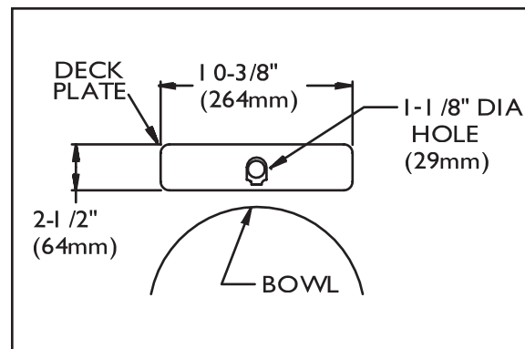
S-8720-CA-E S-8721-CA-E
