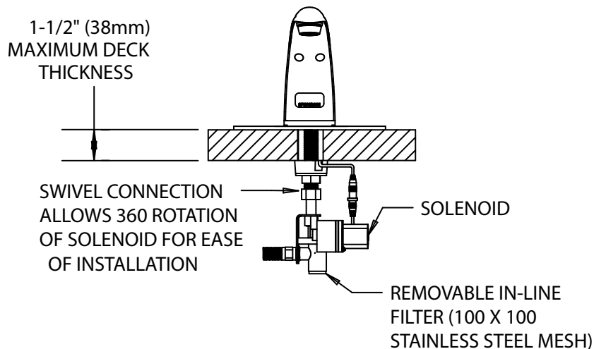
S-8710-CA-E S-8711-CA-E
