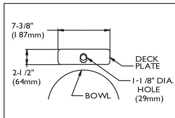
S-8720-CA-E S-8721-CA-E
