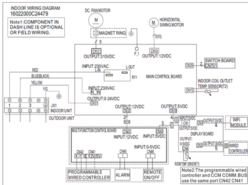
Fig. 17 — Wiring Diagram 6K-12K
