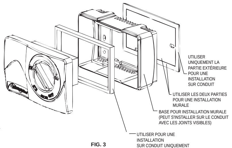
FIG. 3 EMPLACEMENT DU JOINT
