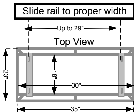
Mini Split Stand (gray) 10" High Part # MIN1832 Pad Size: 24 x 36"
