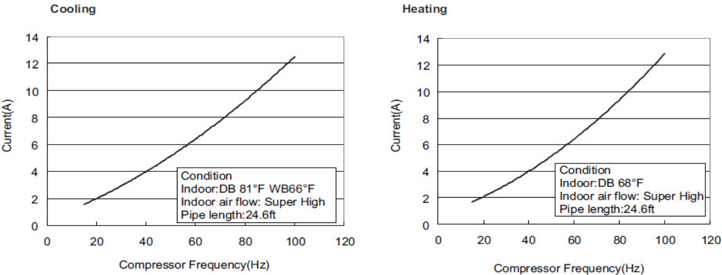
Fig. 8 – 18K
