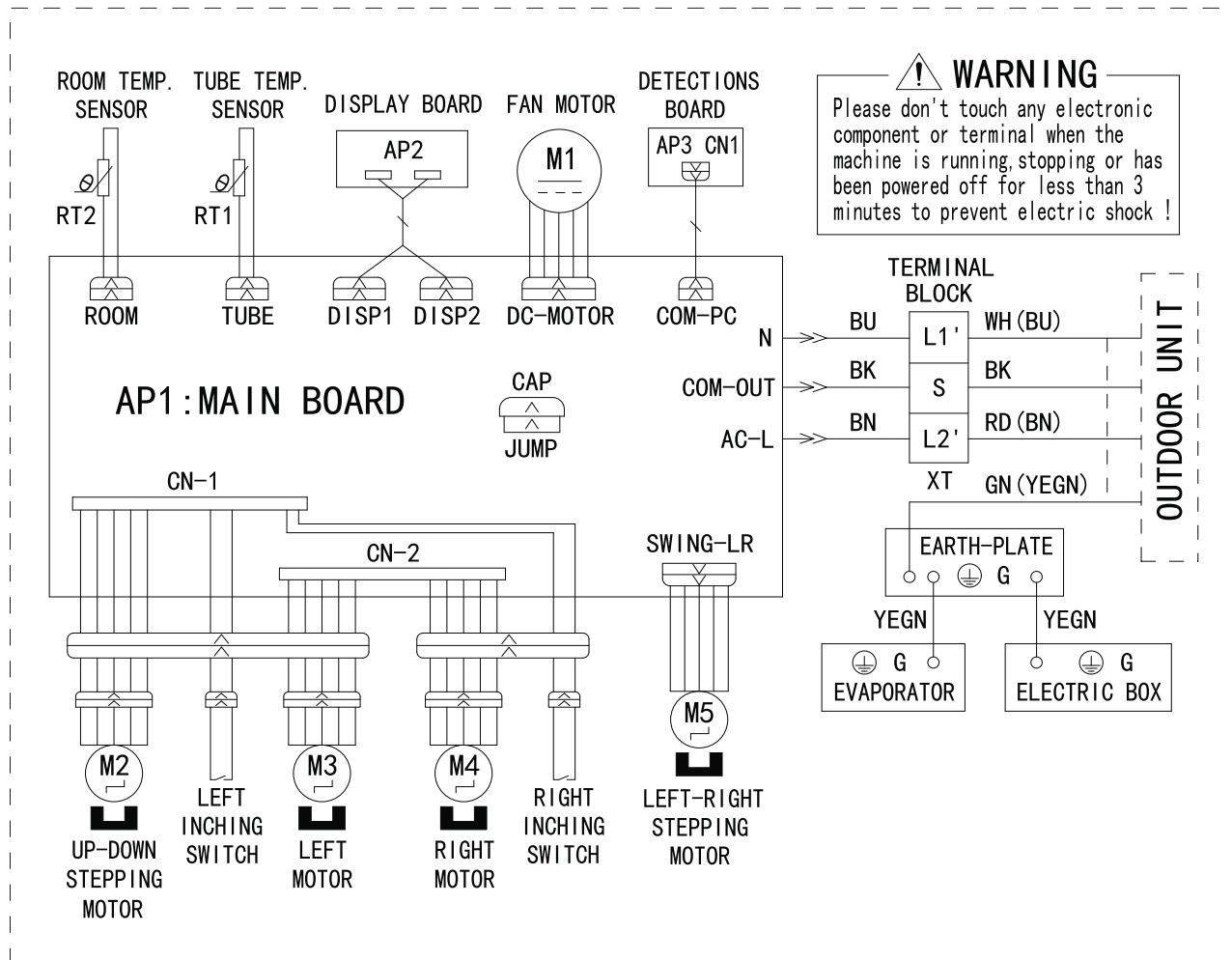
Fig. 13 – Indoor Unit
