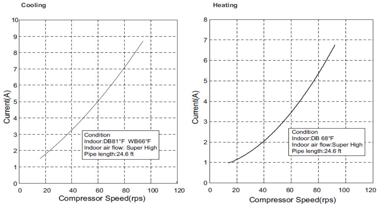
Fig. 7 – 09K/12K
