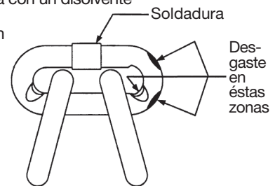
Figura 5a - Inspección de la cadena
