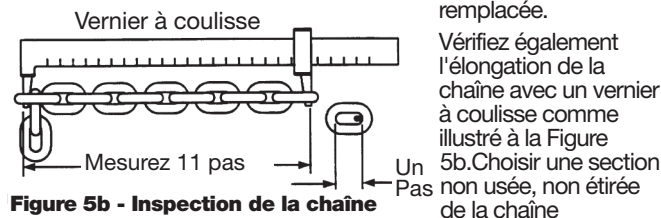
Figure 5b - Inspection de la chaîne
