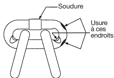
Figure 5a - Inspection de la chaîne
