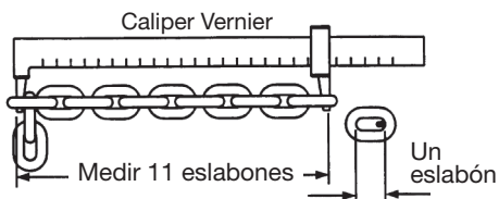
Figura 5b - Inspección de la cadena
