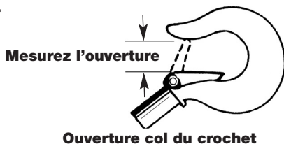
Ouverture col du crochet
