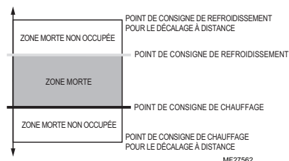
Fig. 26. Commutation automatique avec zones mortes pour les points de consigne de chauffage/refroidissement.
