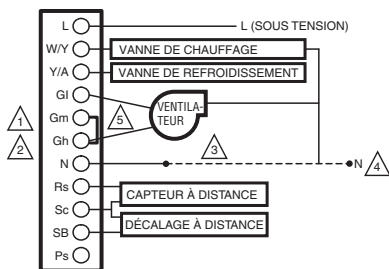
Fig. 12. Schéma de câblage à deux conduits (chauffage ou refroidissement) avec commutation manuelle et chauffage auxiliaire (120/240/277 V c.a. illustré).
