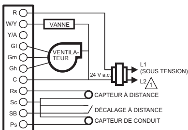
Fig. 17. Schéma de câblage à deux conduits avec commutation automatique (chauffage ou refroidissement) (24 V c.a. illustré).
