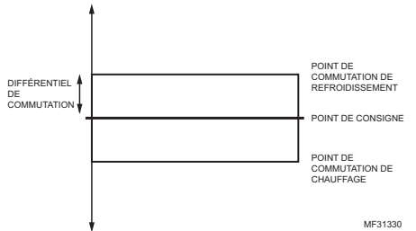
Fig. 29. Système à 4 conduits avec commutation automatique, points de consigne unique et points de commutation.
