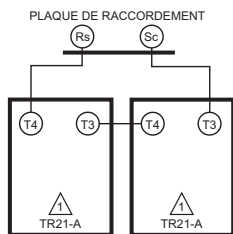
Fig. 5. Câblage de deux capteurs TR21-A (10 K ohms) pour fournir un réseau de moyenne de température.
